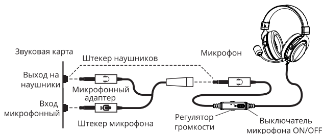
Рис. 2. Схема подключения
